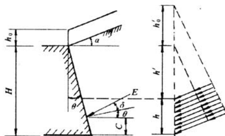
图 A.0.2 主动土压力分层计算图
