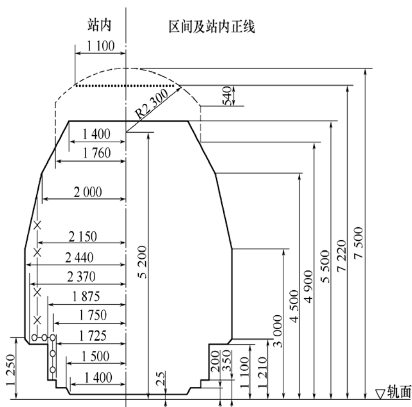
说明图 1.0.10-4 v > 160 km/h 客货共线铁路基本建筑限界轮廓及基本尺寸 (单位: mm)
