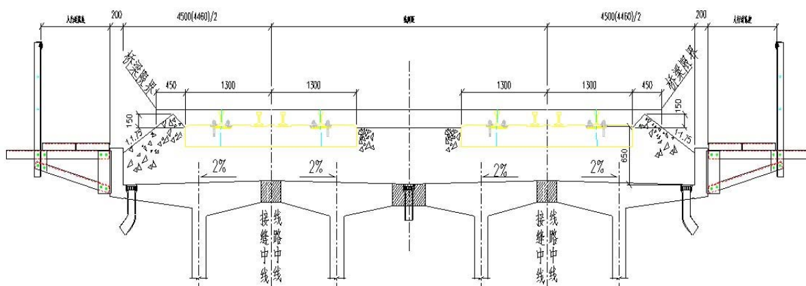
说明图 3.5.1-5 有砟轨道双线直线梁桥面布置图
