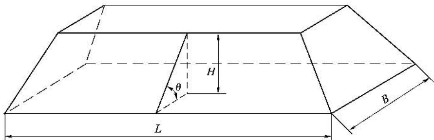
图 A.0.1 梯形台形式堆垛示意图
