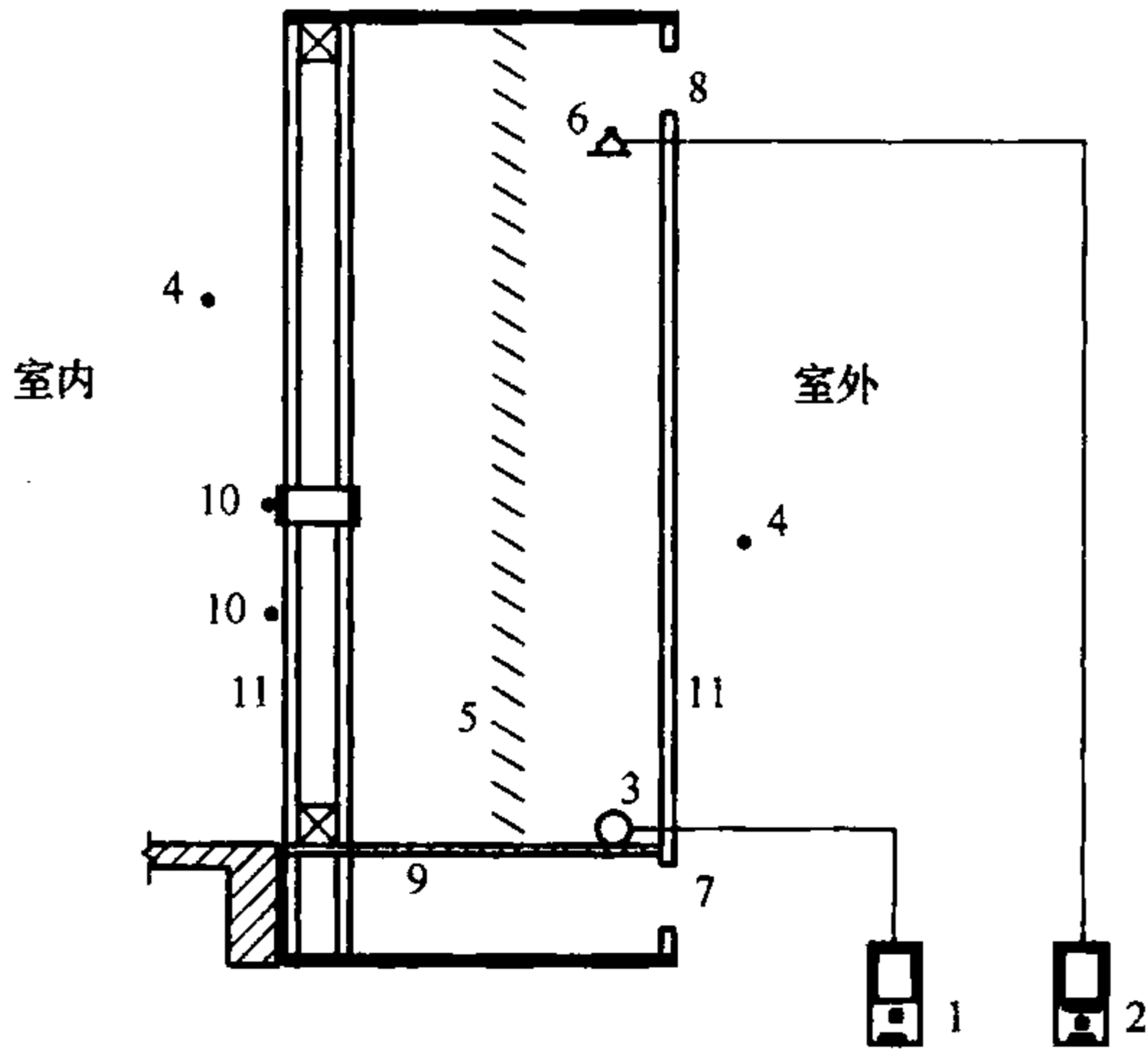
图1 双层幕墙热通道通风量检测系统
