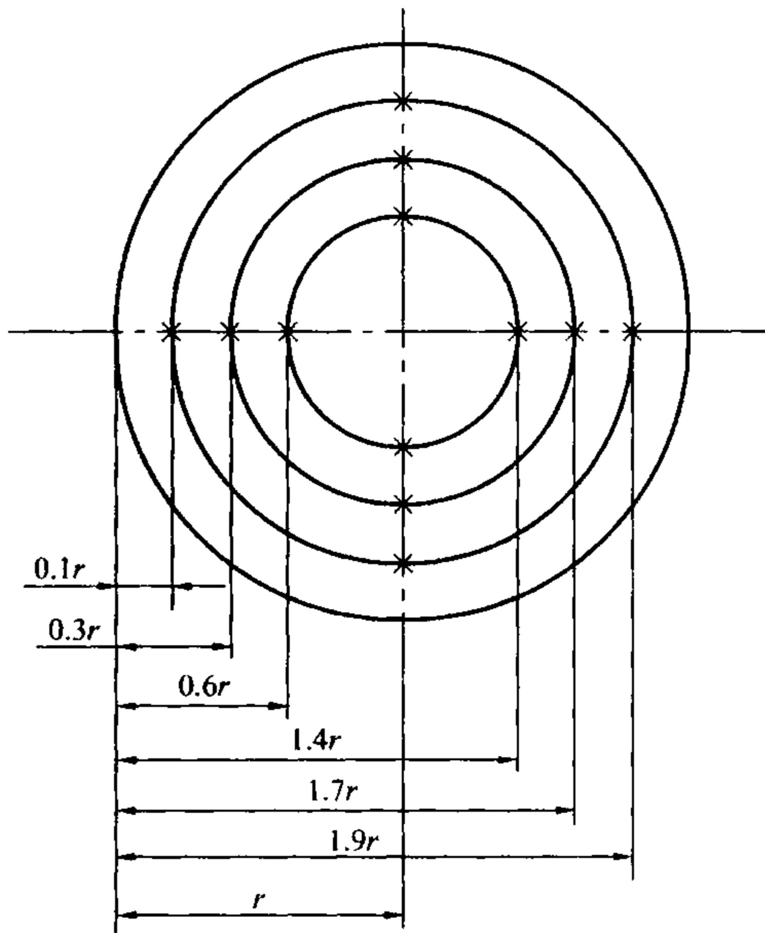
图 E. 1.3-2 圆形风管 3 个圆环时的测点布置
