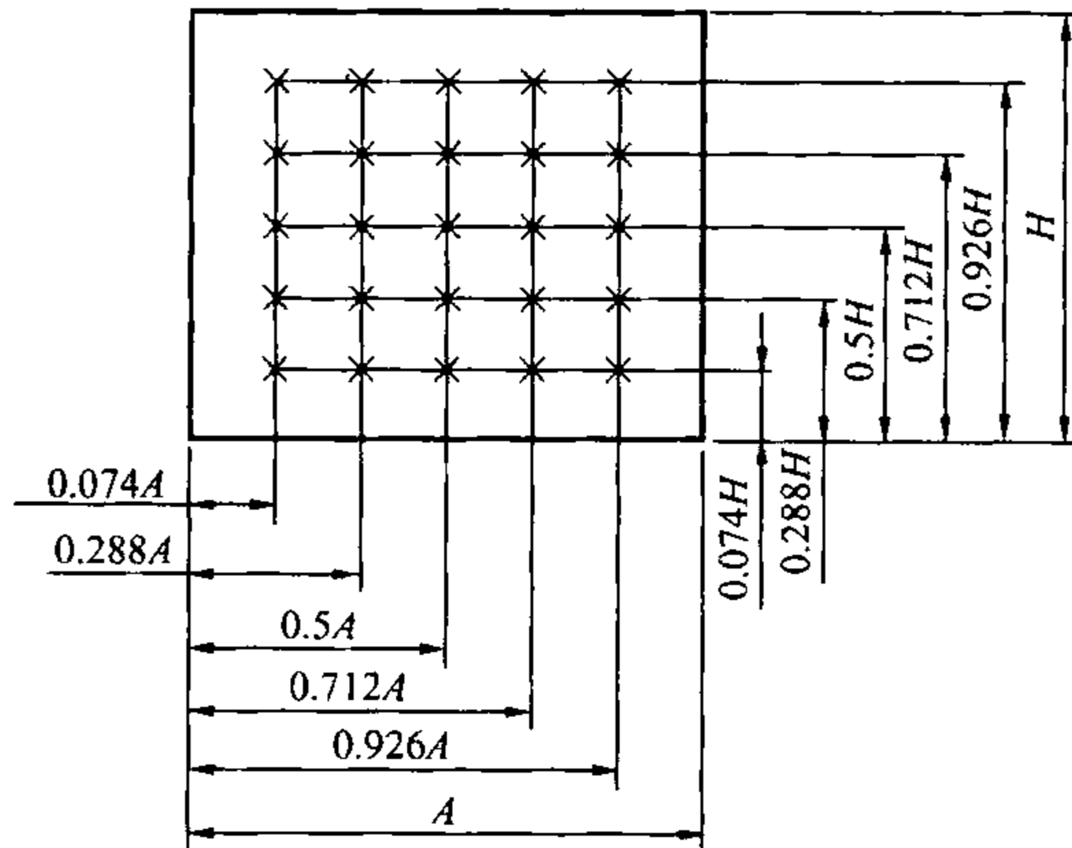
图 E.1.3-1 矩形风管 25 个测点时的测点布置
