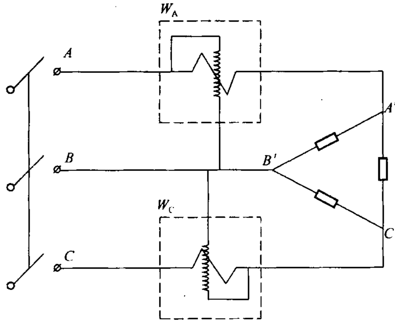
图 2 两表法测量电机输入功率原理
