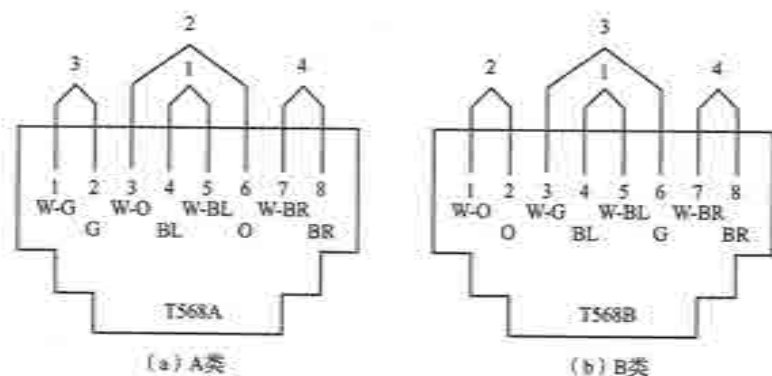
图4.4.4 8位模块式通用插座连接
