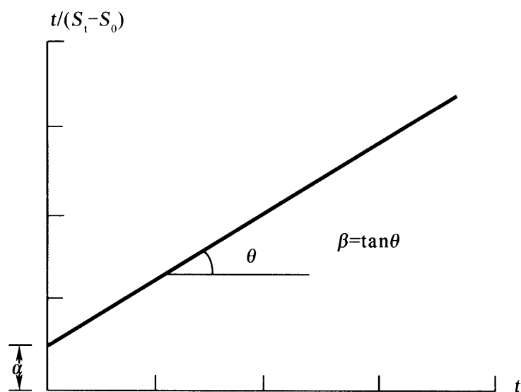
图 B.0.1 \alpha 、 \beta 值确定示意图
