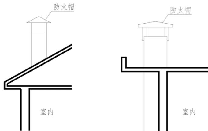
图 9 烟囱防止火星外逸措施示意图
