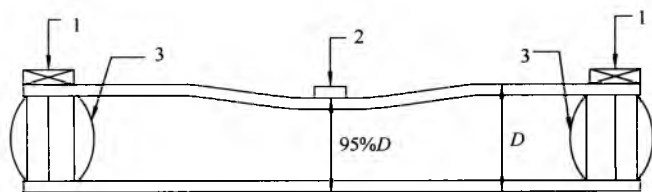
图 B. 2. 4 剪切变形状态下接口严密性测试示意图
