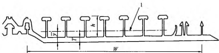
图 10 螺旋缠绕带状型材示意图
