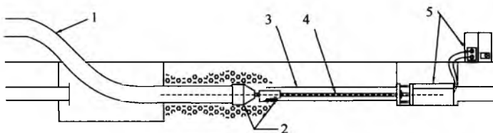
图 15 静拉碎（裂）管法示意图
