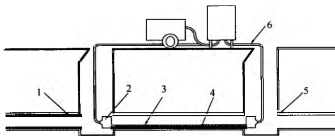
图 13 软管拉入示意图
