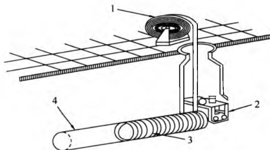
图 6 机械制螺旋缠绕法示意图
