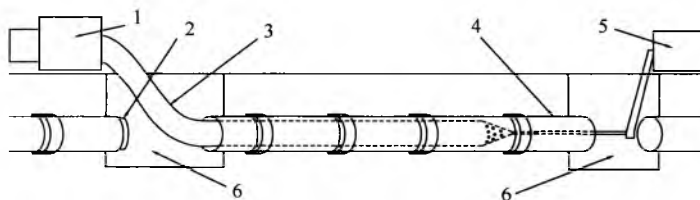
图 5 缩径内衬法示意图
