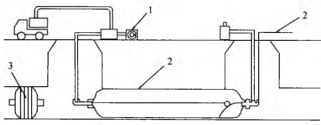
图 3 拉入式原位固化法示意图
