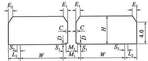
a)高速公路、一级公路(整体式)
