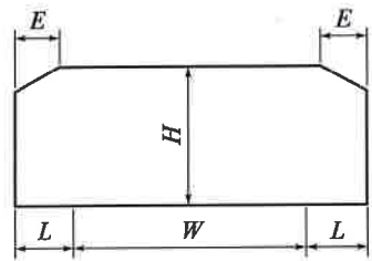
c)二、三、四级公路
