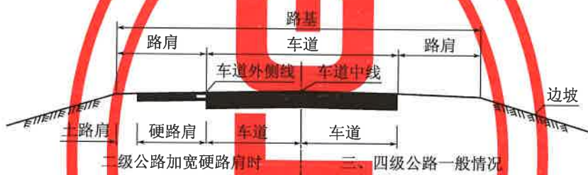
图 4-6 二、三、四级典型断面形式示意图
