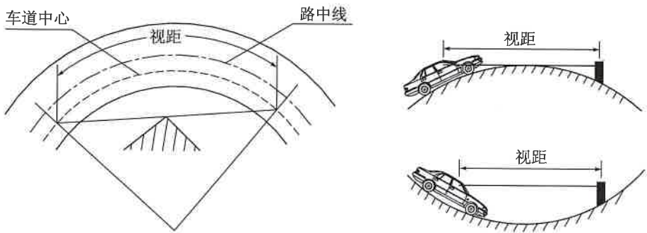
图 4-7 公路平面视距和纵面视距示意图
