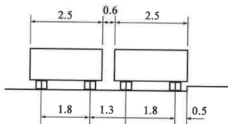
图 7.0.5 车辆荷载横向布置 (尺寸单位:m)
