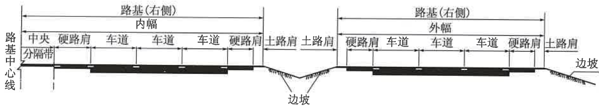
图 4-4 高速公路复合式断面形式示意图（内、外幅路基分离）
