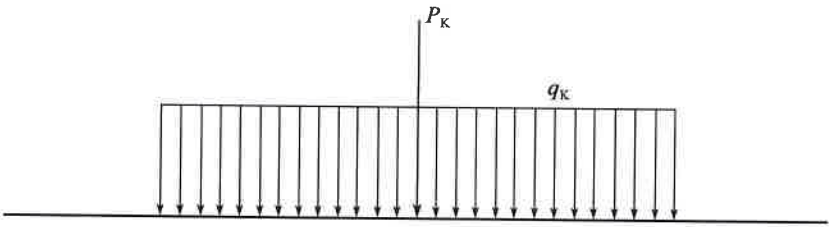
图 7.0.3 车道荷载
