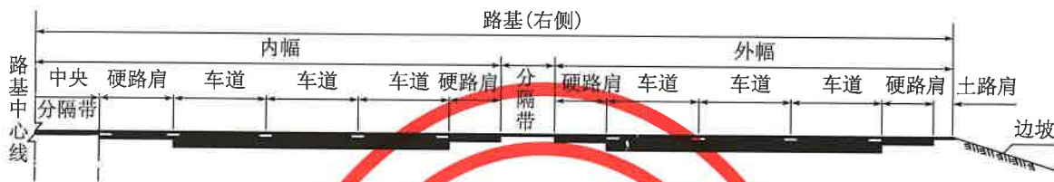
图 4-5 高速公路复合式断面形式示意图（内、外幅整体式）
