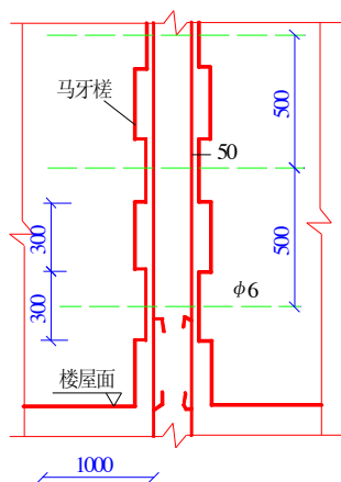
图 5.3.3-1 拉结钢筋布置及马牙槎示意图
