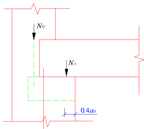
图 4.1.5 梁端支承压力位置
