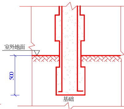
图 5.3.3-2 构造柱根部示意图
