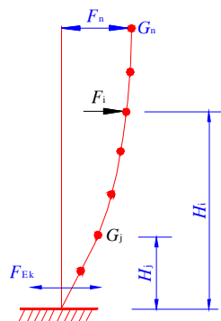
图 5.2.5 结构水平地震作用计算简图
