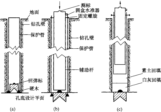
图 29 辅助杆压入式标志埋设步骤
