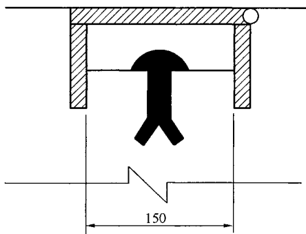
图 33 盒式标志 (适用于设备基础上埋设, 单位: mm)
