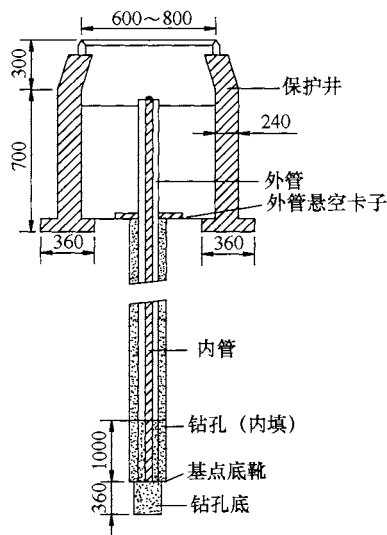
图 13 深埋钢管水准基点标石 (单位: mm)
