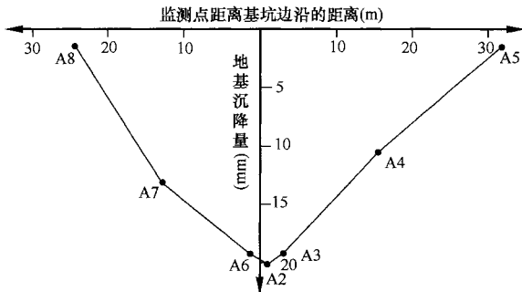
图 22 相邻地基沉降的距离-沉降曲线
