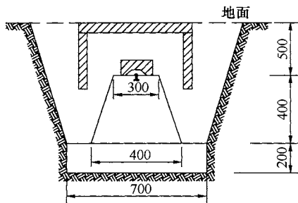
图 16 混凝土普通水准标石 (单位: mm)
