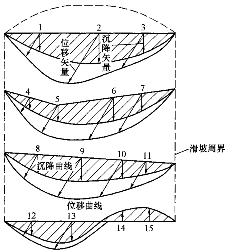
图 28 某斜坡监测点位移综合曲线图
