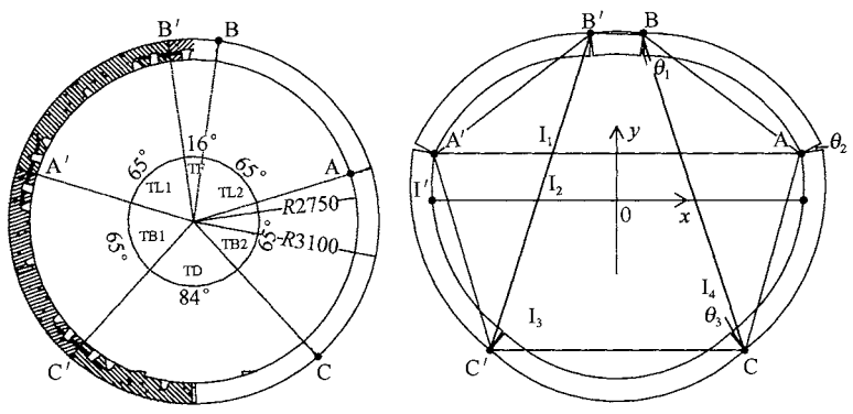
图 39 典型的收敛变形示意图
