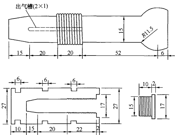
图 34 螺栓式标志 (适用于墙体上埋设, 单位: mm)
