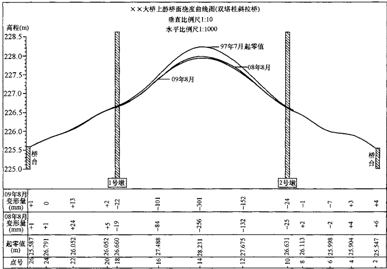
图 38 挠度曲线
