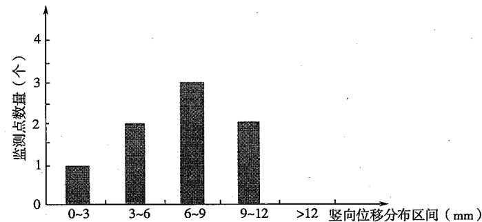
图1 桩顶竖向位移数据统计
